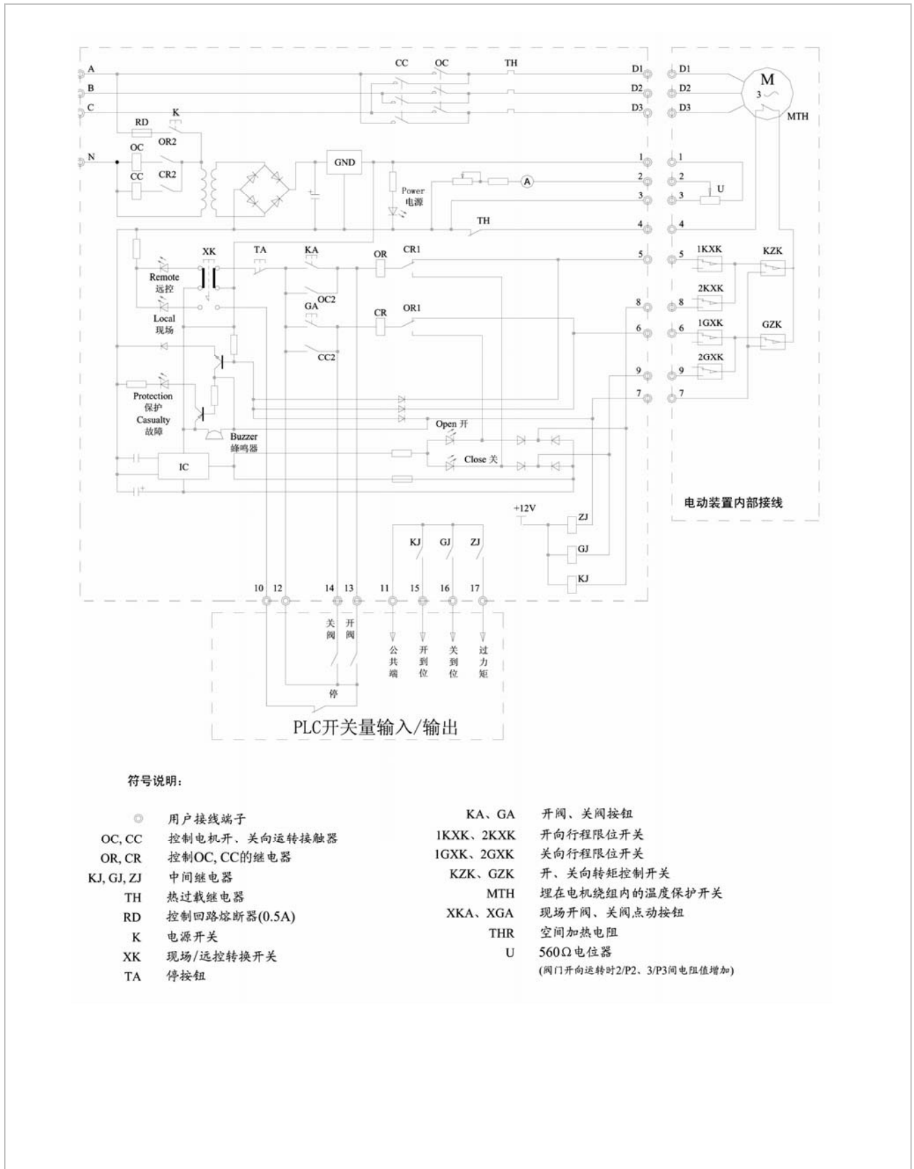
DFK-1C / DFK-2C 型电动阀门控制器 电气原理图
